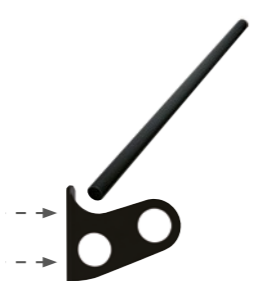
Wspornik do rur śniegowych Rura śniegowa Ø 40 Funkcja: 4080/4090
