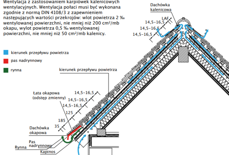
Rysunek techniczny produktu AMBIENTE KRÓJ SEGMENTOWY - przekrój wzdłużny połaci dachu
